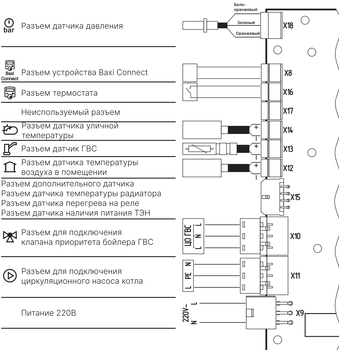
Рис.10 Схема подключения датчиков «X-Line100E»
