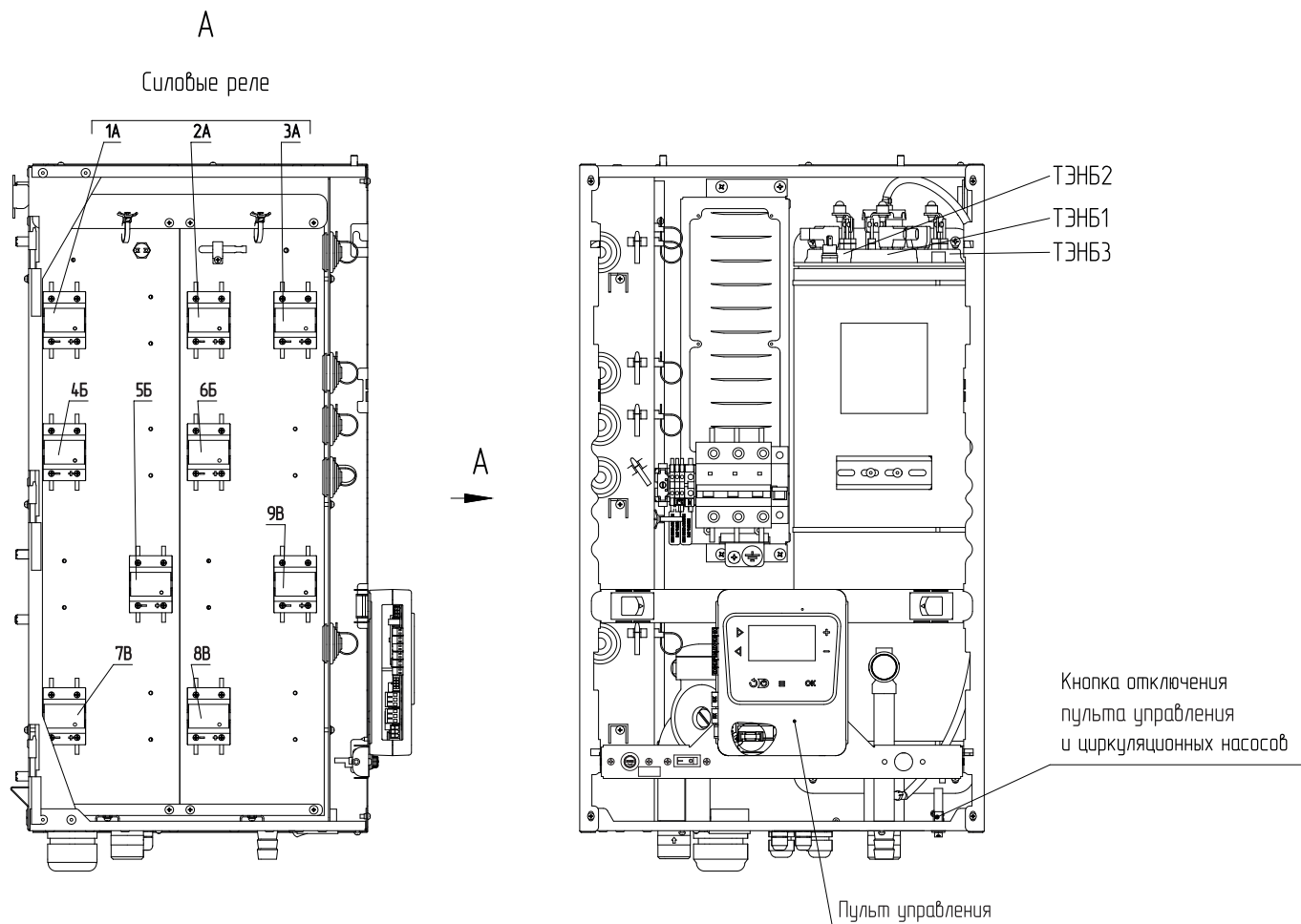
Рис.13 Органы управления электрического котла BAXI Ampera Pro 30-45 кВт
