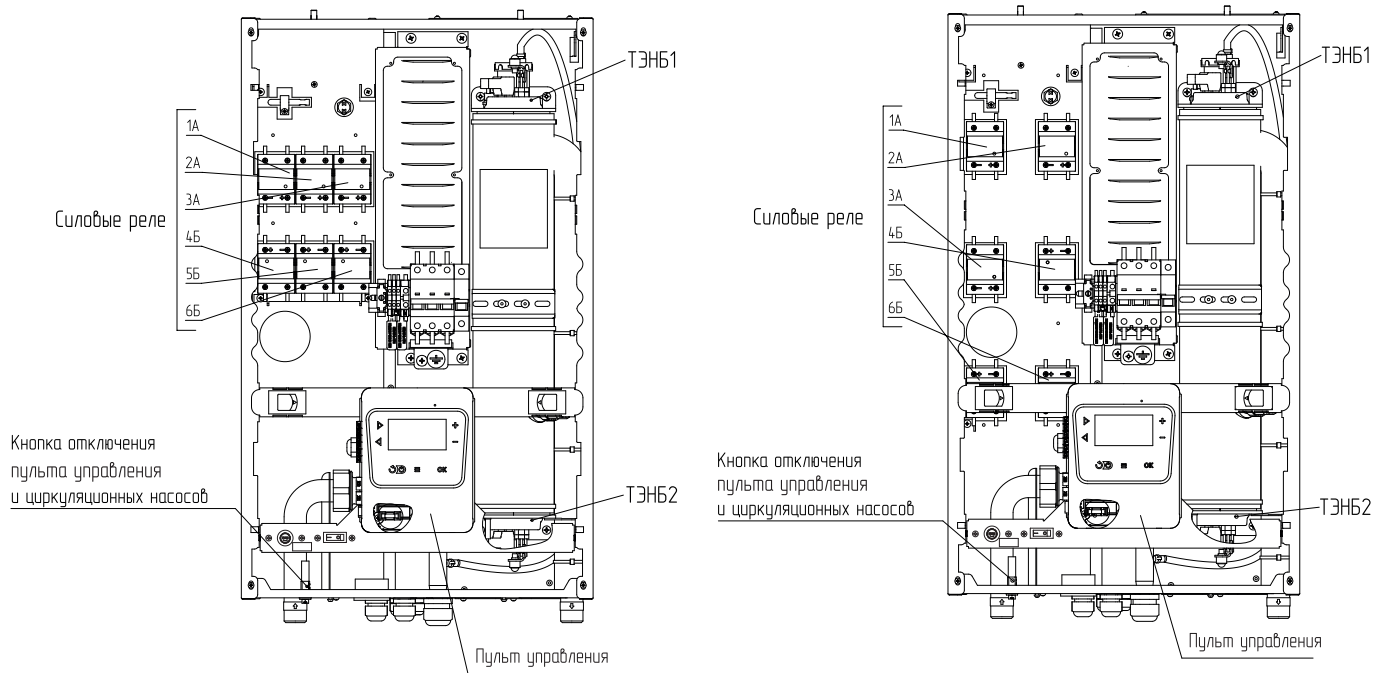
Рис.12 Органы управления электрического котла BAXI Ampera Pro 9-24 кВт
