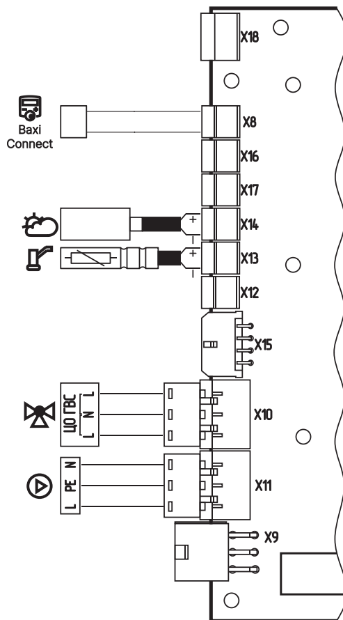
Рис.18 Подключение клапана приоритета бойлера ГВС, датчиков ГВС и улицы, к контроллеру «X-Line 100E»
