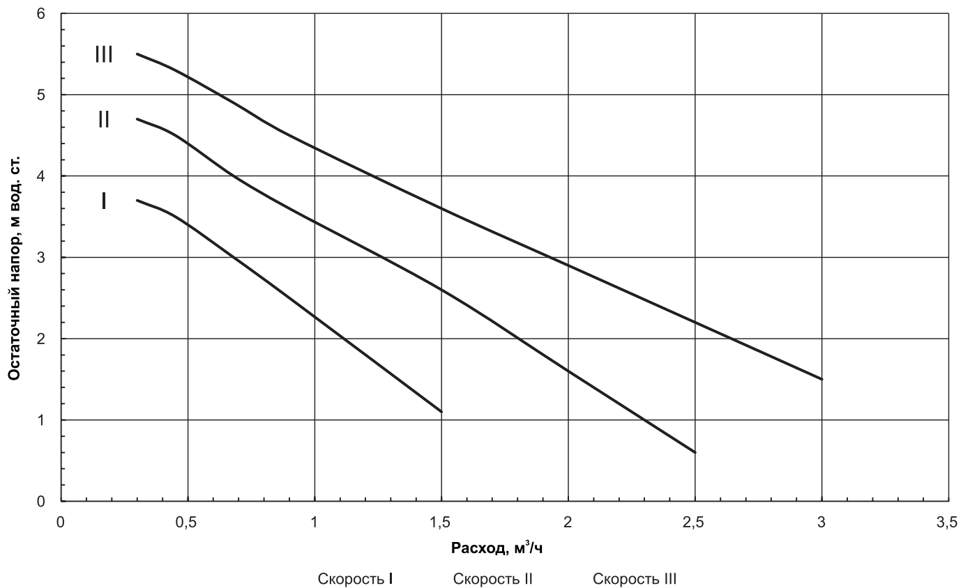
Рис.22.1 Напорные характеристики циркуляционного насоса 25/70 котлов BAXI AMPERA Pro 30-45 кВт
