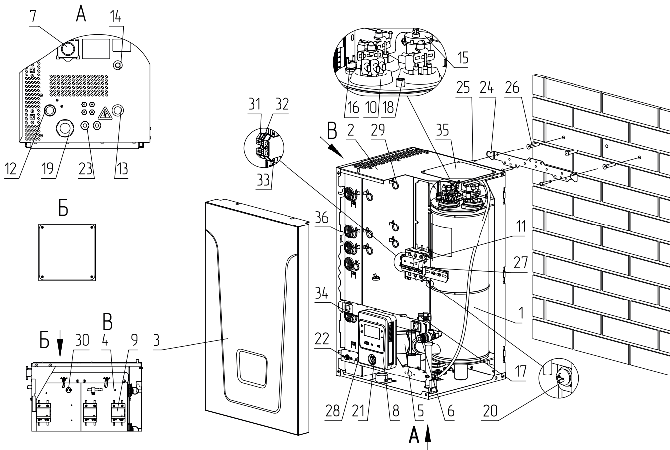
Рис.2 Конструкция котла
