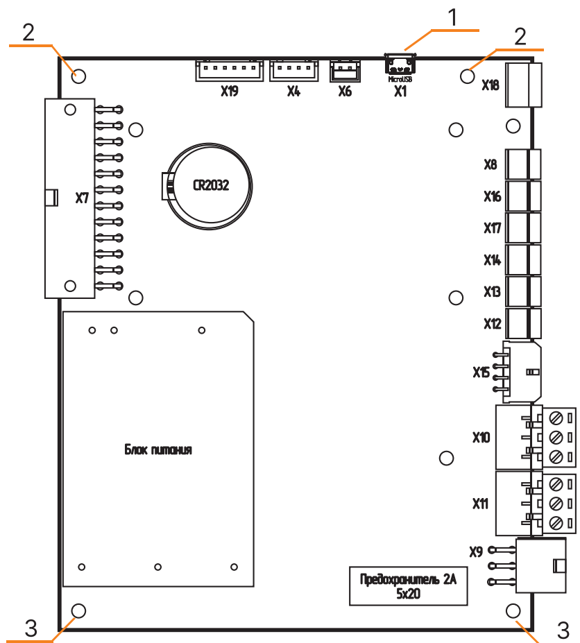
Рис.26 Плата контроллера
