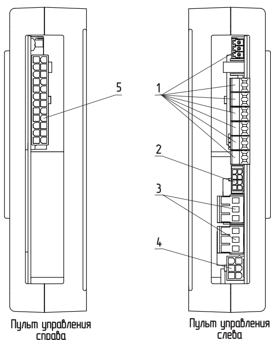
Рис.11 Расположение и назначение разъемов контроллера «X-Line100E»
