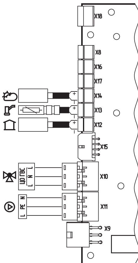
Рис.17 Подключение клапана приоритета бойлера ГВС, датчиков температуры в помещении, ГВС и улицы к контроллеру «X-Line 100E»
