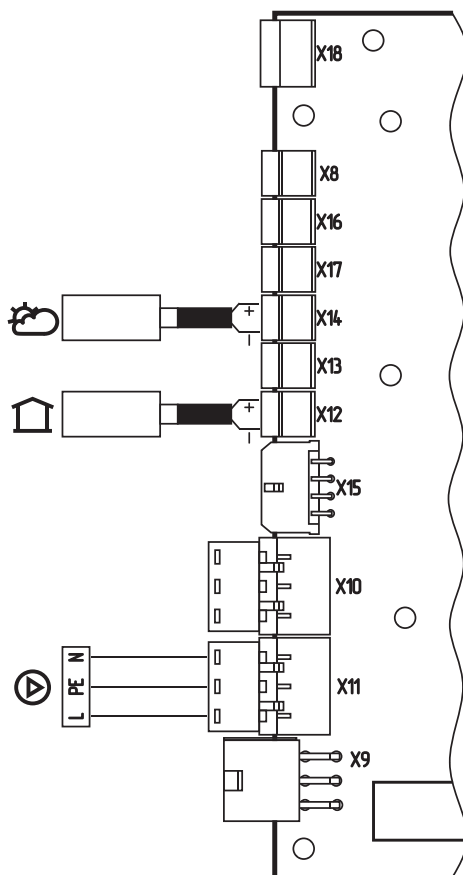
Рис.16 Подключение датчиков температуры в помещении и улицы к контроллеру «X-Line 100E»
