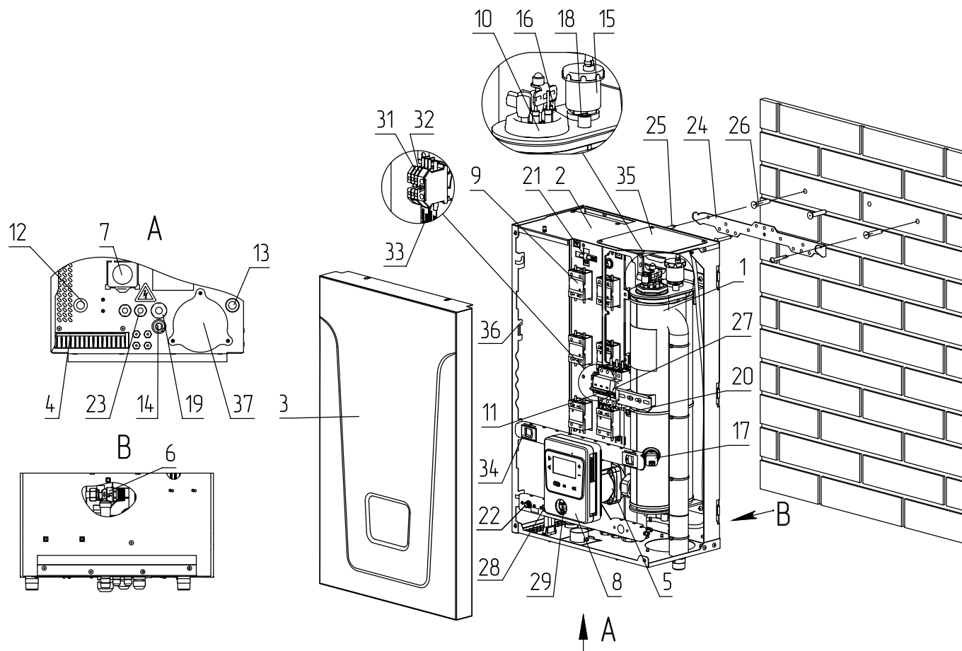
Рис.1 Конструкция котла
