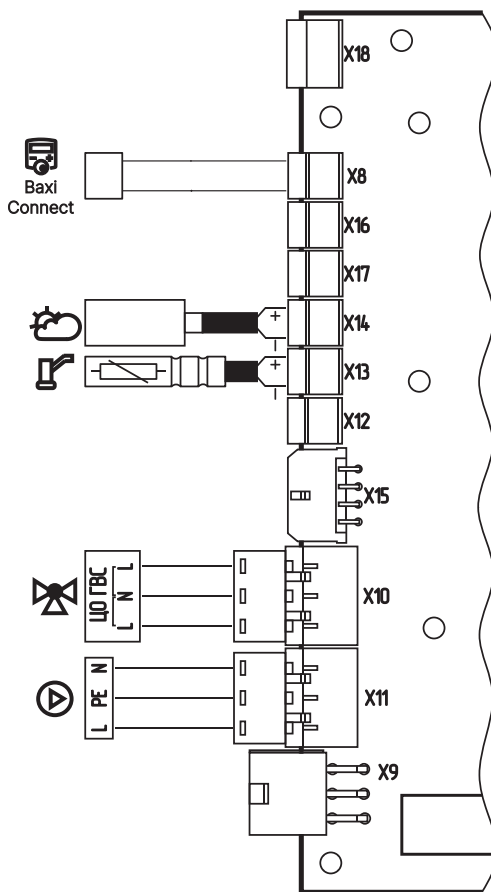
Рис.19 Подключение клапана приоритета бойлера ГВС, датчиков ГВС и улицы, и устройства Baxi Connect к контроллеру «X-Line 100E»
