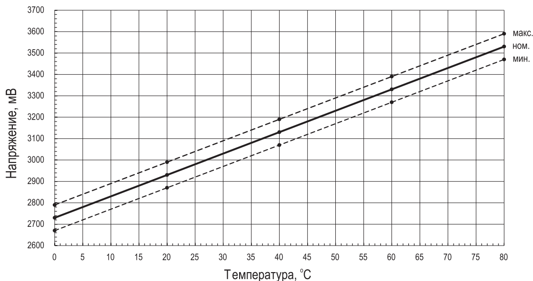
Рис.21 Напряжение на датчике в зависимости от температуры
