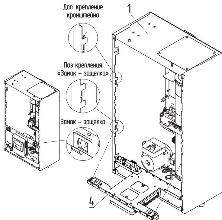
Рис.7 откидывание кронштейна
