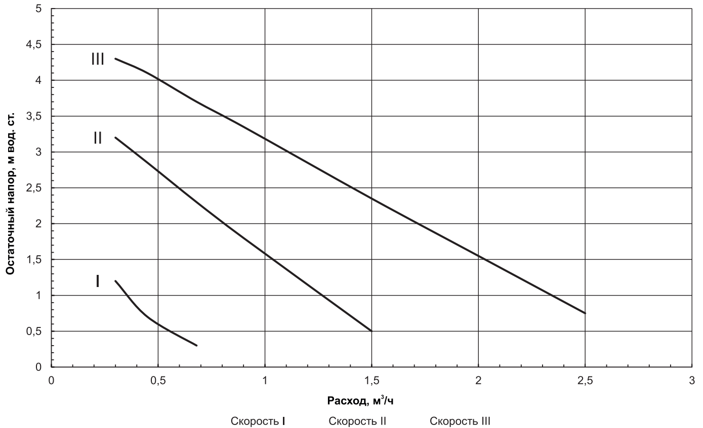
Рис.22 Напорные характеристики циркуляционного насоса 25/60 котлов BAXI AMPERA Pro 12-24 кВт
