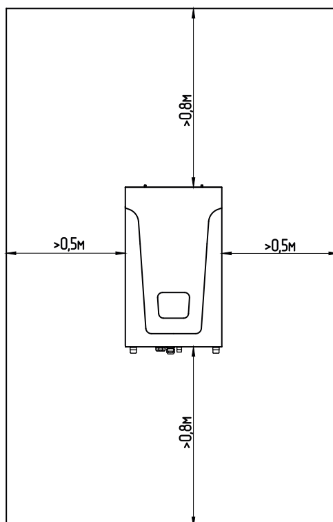
Рис.3 Схема размещения котла в котельной
