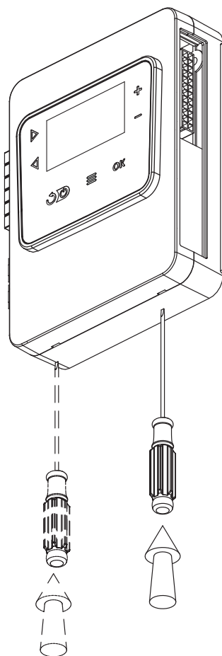
Рис.25 Демонтаж лицевой панели
